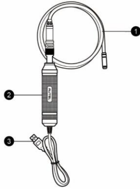
图 15-1 高清内窥镜
